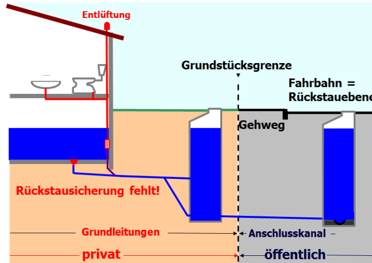
Abbildung 1: Überflutung des Kellers bei Rückstau im Schmutzwasserkanal durch eine fehlende Rückstausicherung im Bodenablauf des Kellers.
