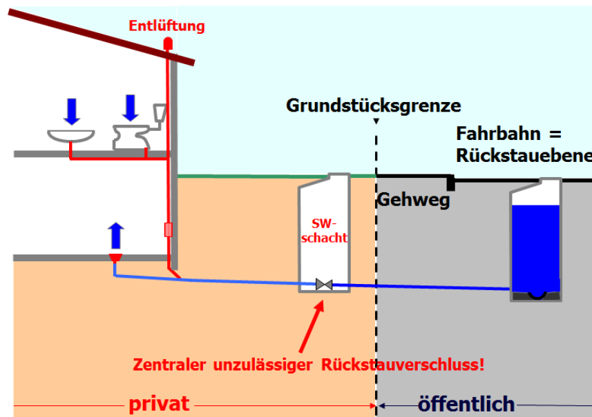
Abbildung 3: Überflutung des Gebäudes durch einen zentral geschlossenen Rückstauverschluss
