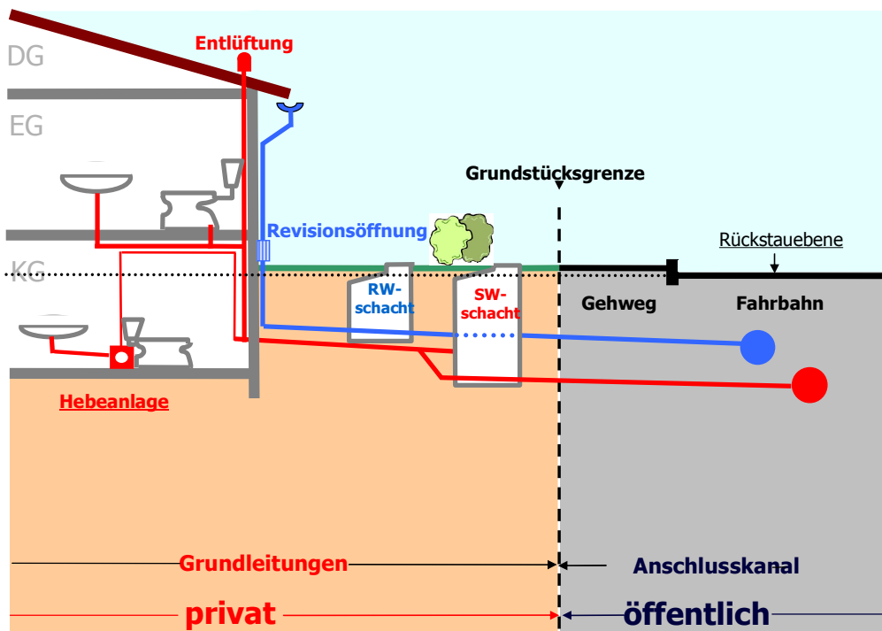
Abbildung 2: Rückstausicherung eines Hauses über Hebeanlage
