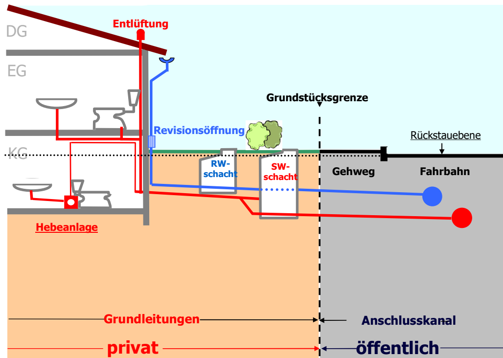
Abbildung 2: Rückstausicherung eines Hauses über Hebeanlage
