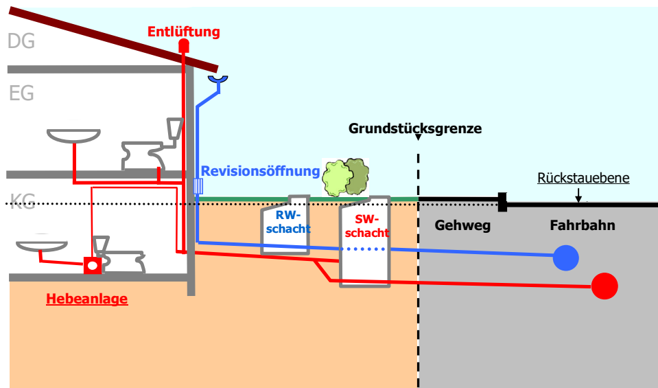
Abbildung 2: Rückstausicherung eines Hauses über Hebeanlage
